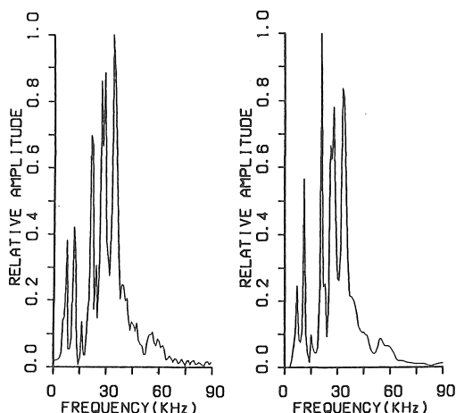
図-2 周波数応答 (伝播解析結果)
