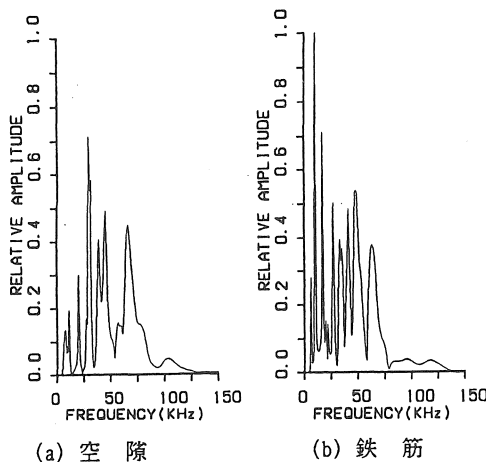
図-9 周波数応答 (直径=40mm、かぶり厚さ=51mm、間隔=5.2cm)
