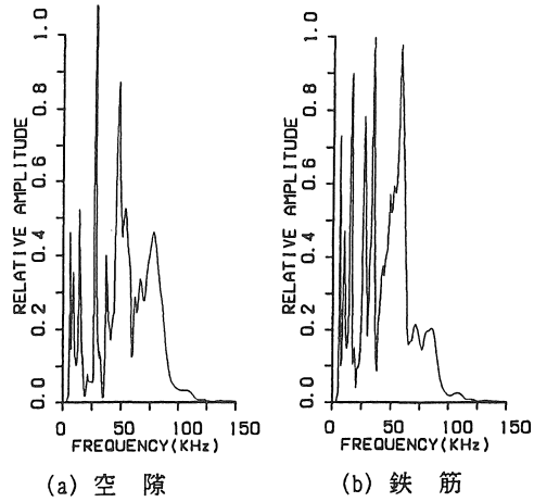
図-10 周波数応答 (直径=22mm、かぶり厚さ=69mm、間隔=7cm)
