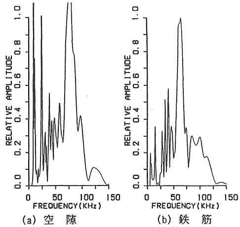
図-8 周波数応答 (直径=40mm、かぶり厚さ=9mm、間隔=5cm)
