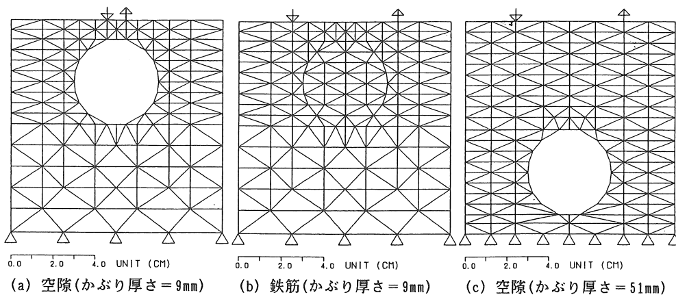
図-1 解析モデルの概要
