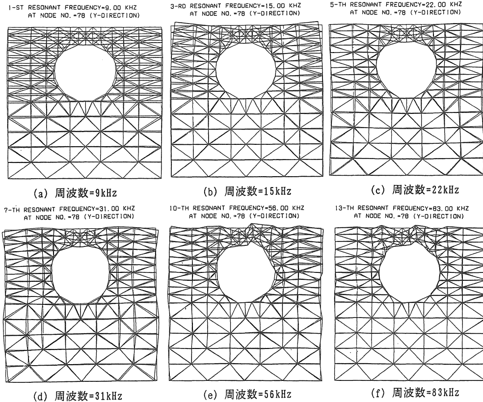
図-5 低周波数領域の振動モード例 (介在物=空隙、直径=40mm、かぶり厚さ=9mm、間隔=0.9cm)
